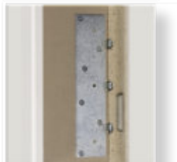
verstärktes Schließblech mit Stahlhalteplatte Nr. 35 Ansicht Futterrückseite
