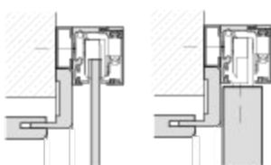
Montage mit DUFU mit Distanzprofil
